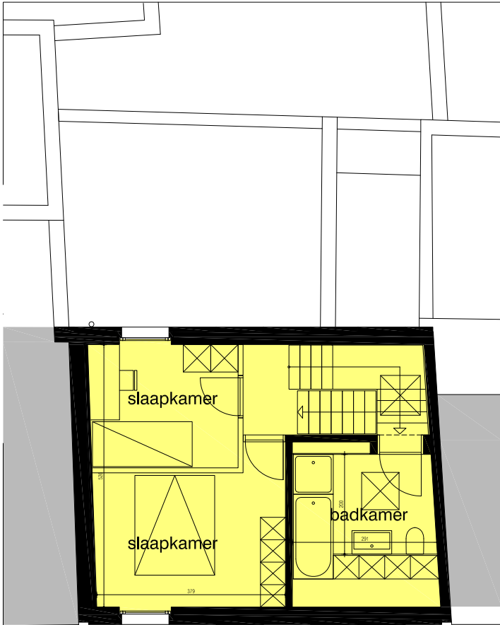
Tweede verdieping
