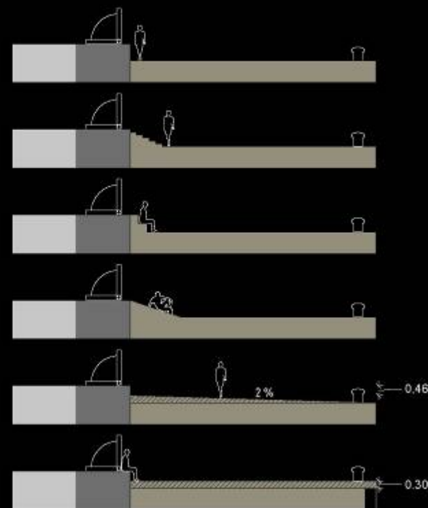
overgang waterkering / kaaien
