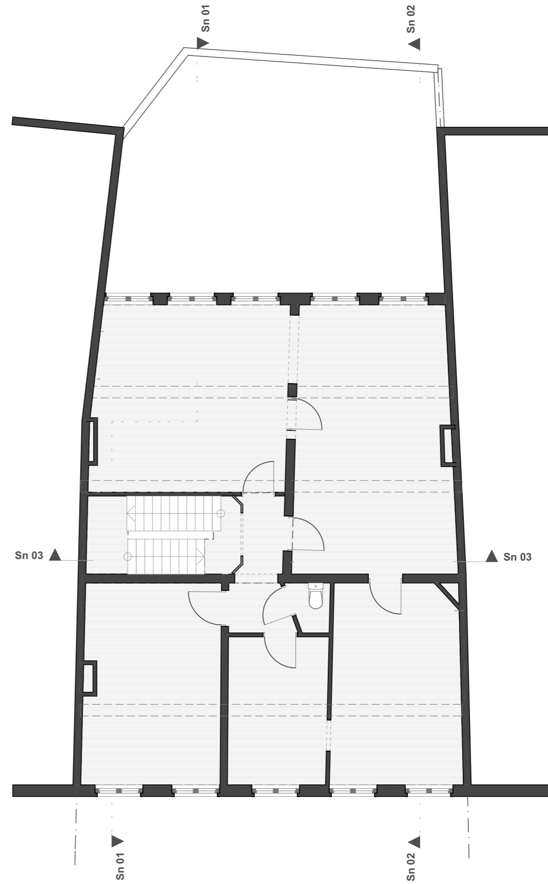
2. 2e Verdieping
