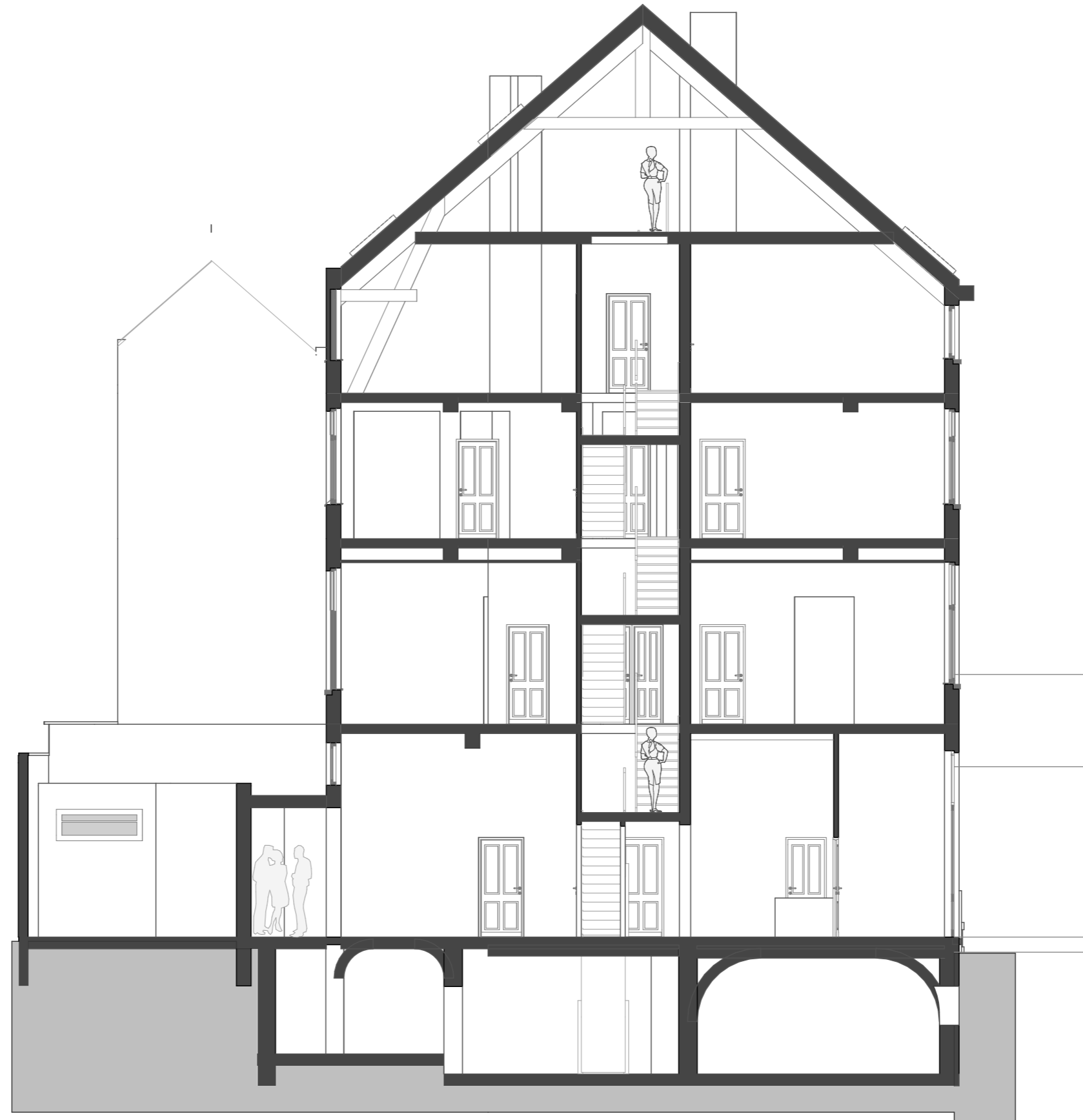
Sn 01
