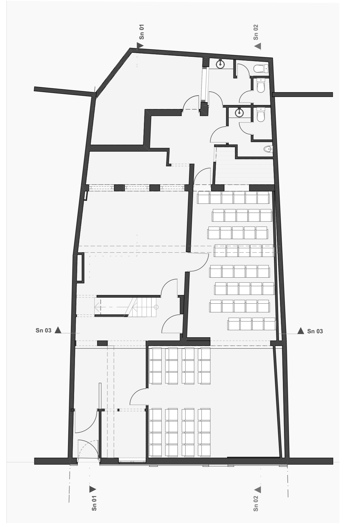
0. Gelijkvloers
