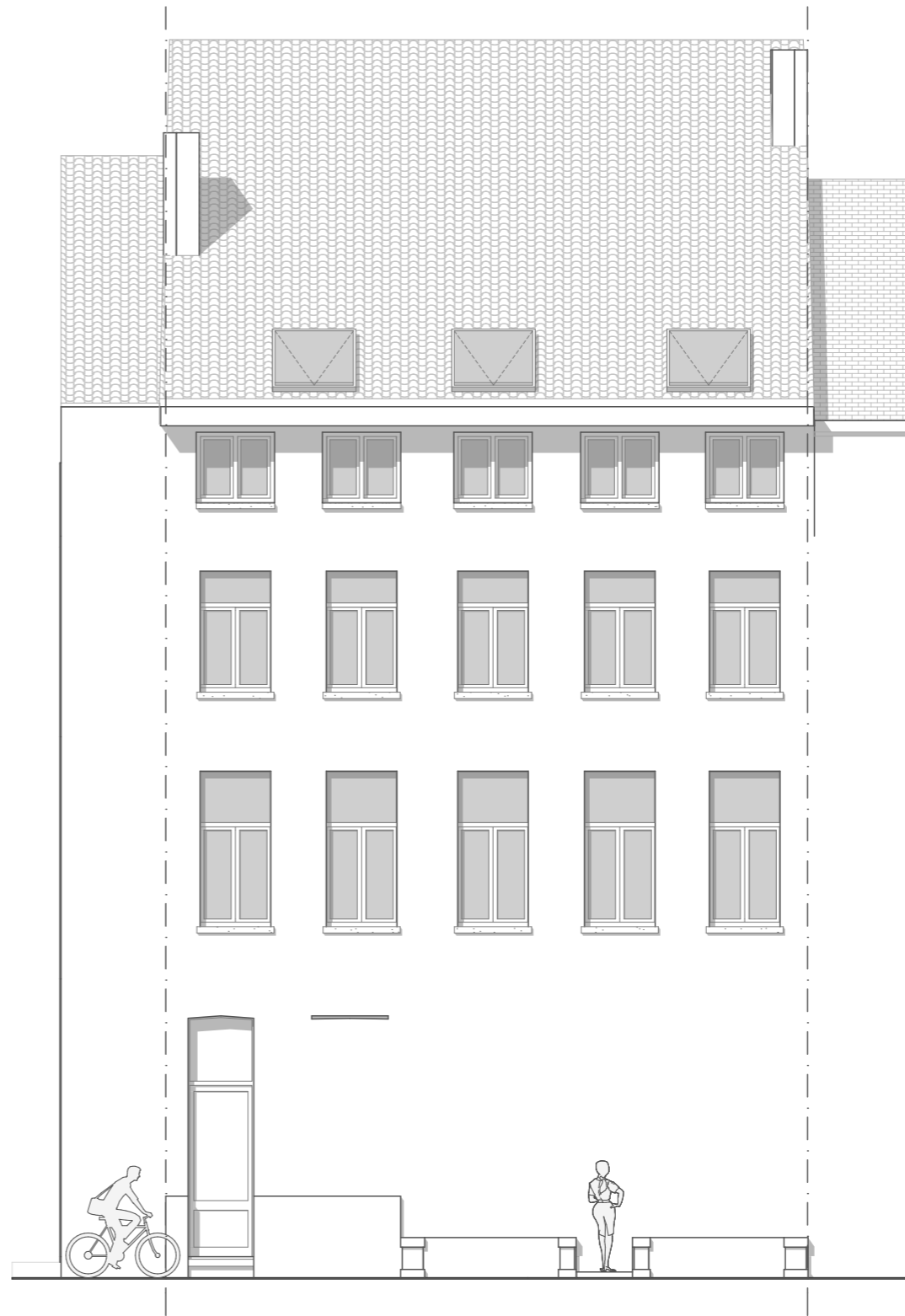
GV VOORGEVEL
