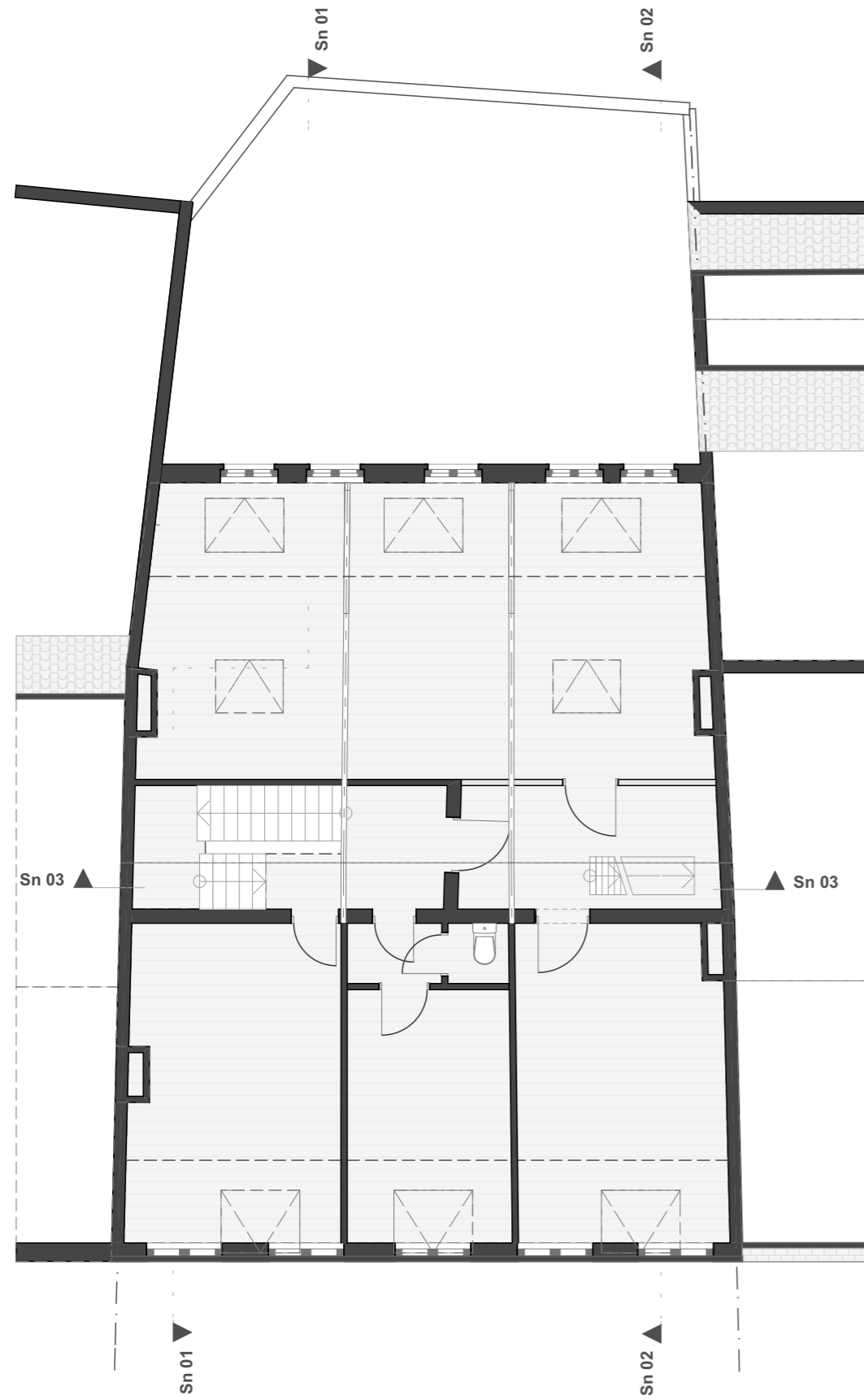
3. 3e Verdieping
