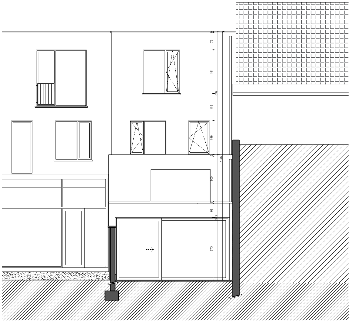
ACHTERGEVEL
