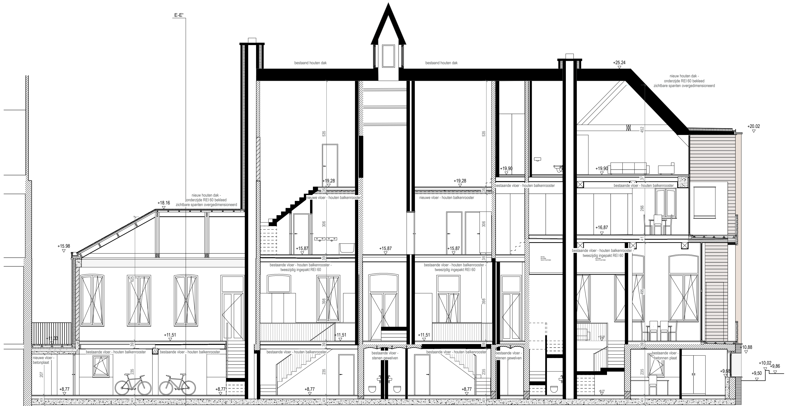
Doorsnede F-F'
