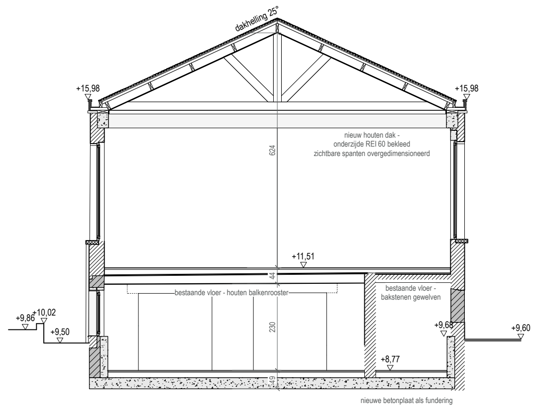
Doorsnede E-E'
