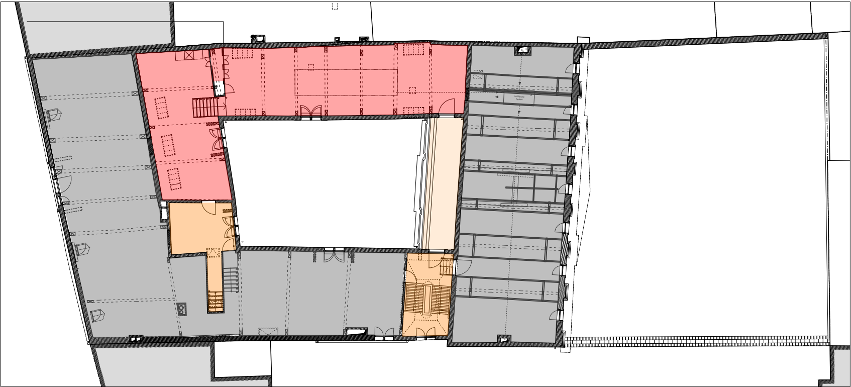
Tweede verdieping/zolder - schaal 1:250
