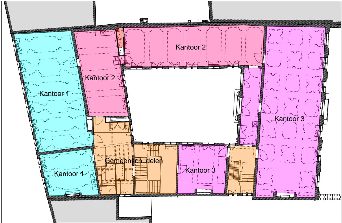
Eerste verdieping - schaal 1:250
