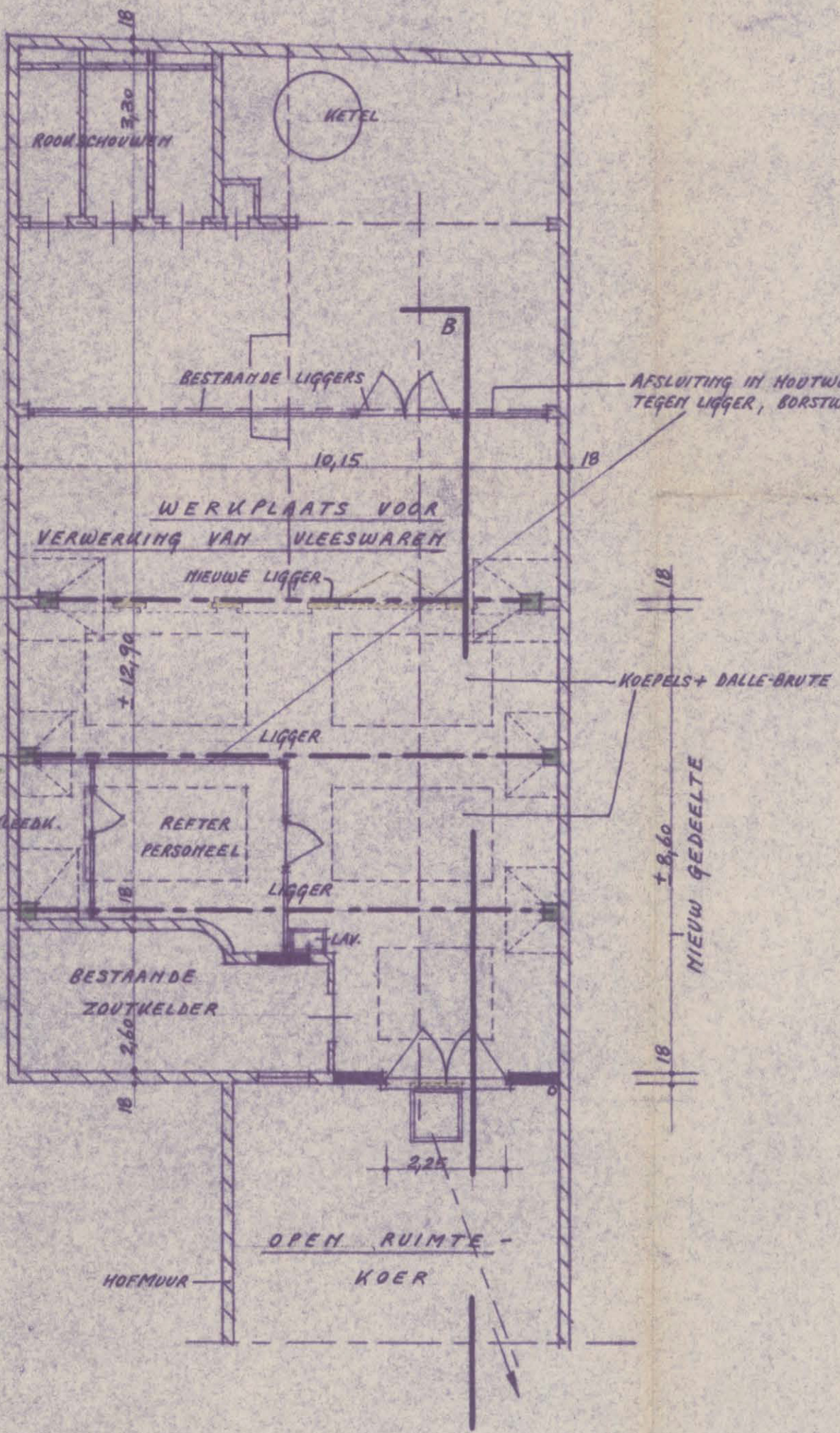
WERKPLAATS OP 1 CM. PER M.
